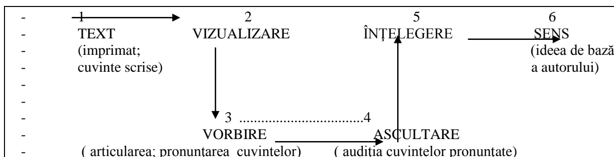
Fig. 1. Procesul citirii
